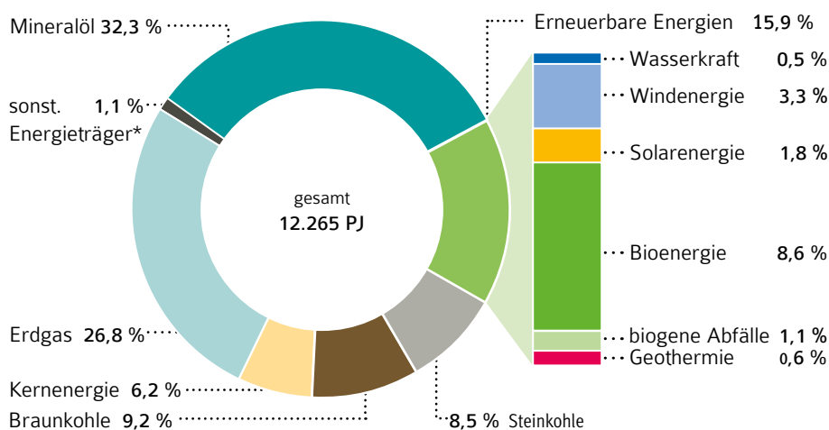
Abb. 4: Primärenergieverbrauch 2021
